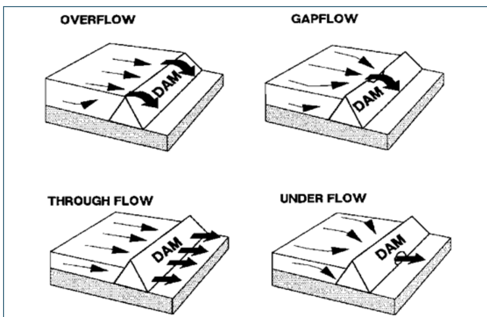
Abb. 3: Schematische Darstellung der vier verschiedenen Abflusstypen
